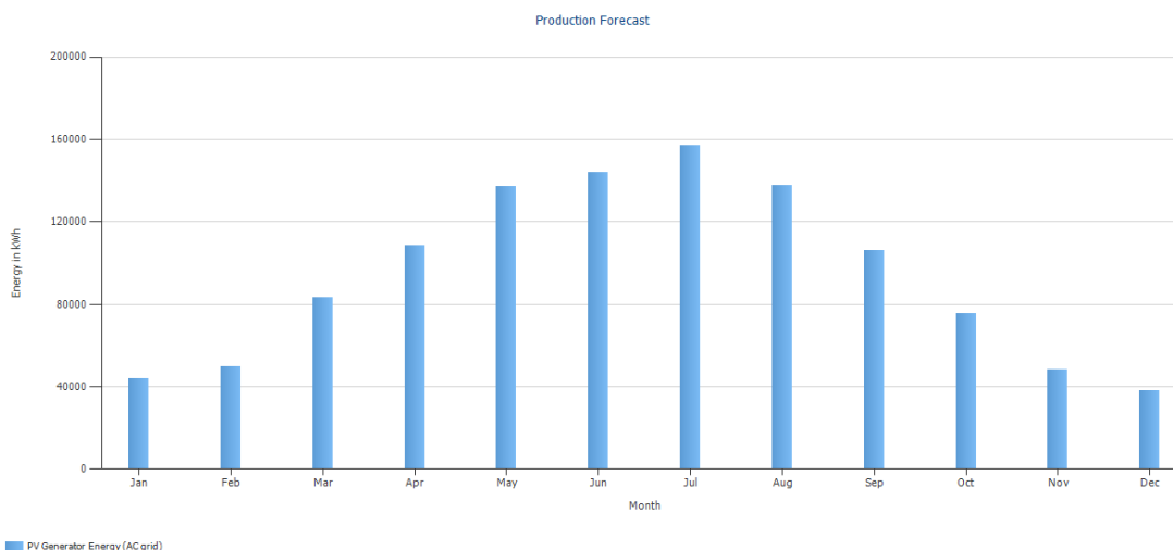
Slika 5: Očekivana mjesečna proizvodnja električne energije iz predložene fotonaponske elektrane, izražena u kWh
